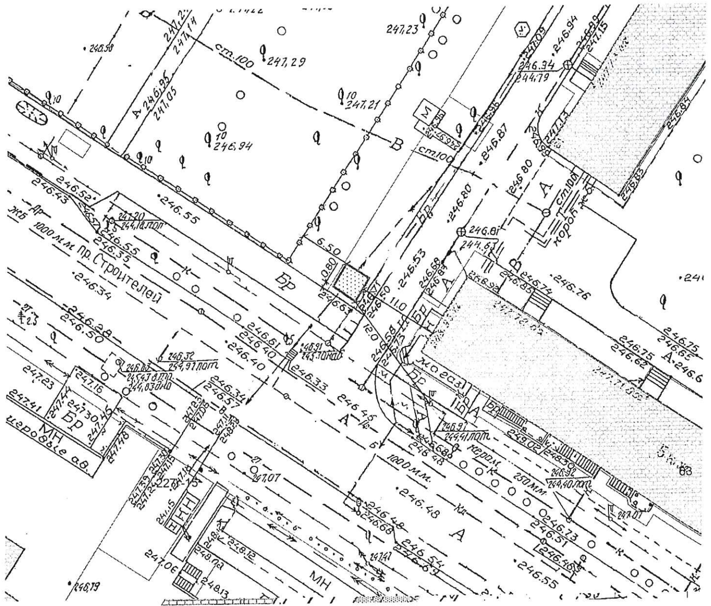
Топографическая основа в масштабе 1:500
