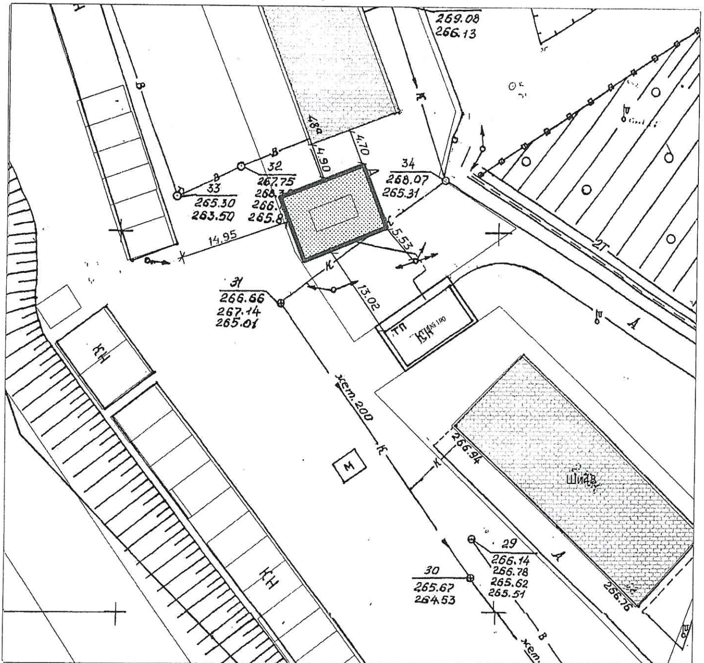
Топографическая основа в масштабе 1:500
