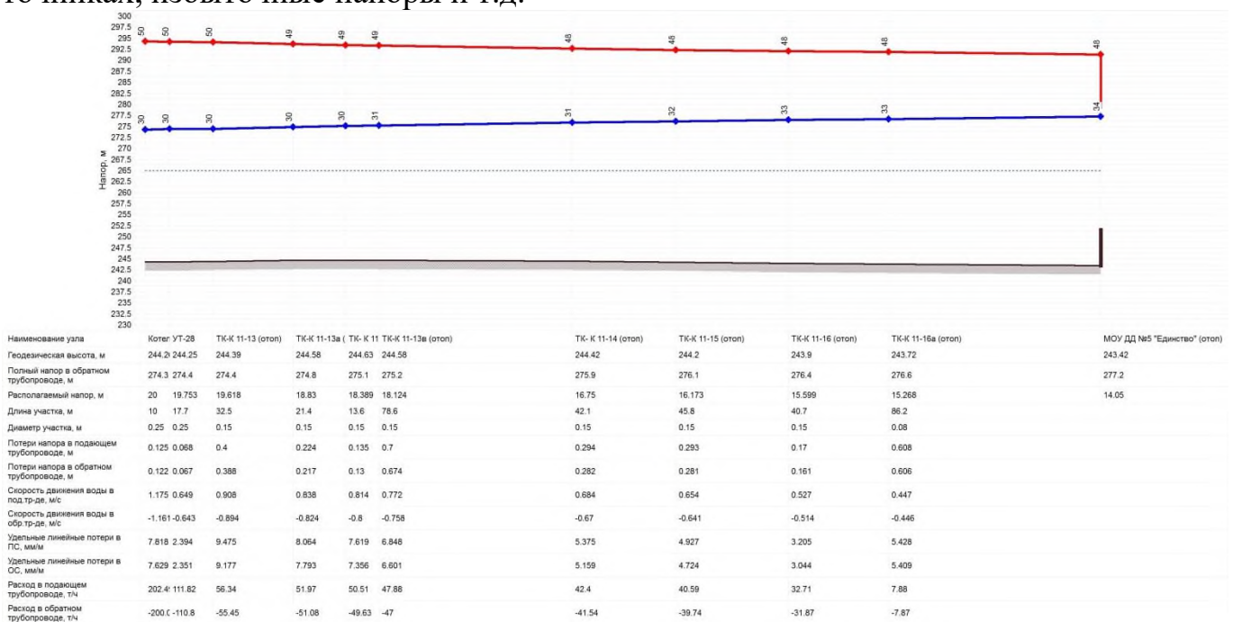
Рис. 12. Пьезометрический график
