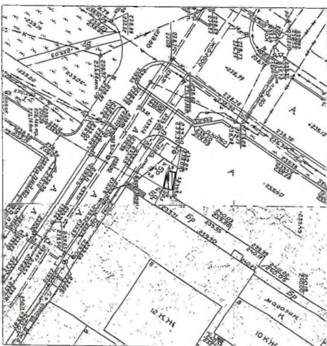
Топографическая основа в масштабе 1:500
